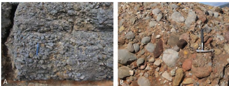
Exemples de conglomerats grisencs de Collegats, amb còdols d'àrea font cretàcia (A) i de conglomerats vermellosos de Montsor, amb còdols d'origen paleozoic i permotriàsic (B). Fotografies d'Alex Whittaker (Imperial College, Londres).
