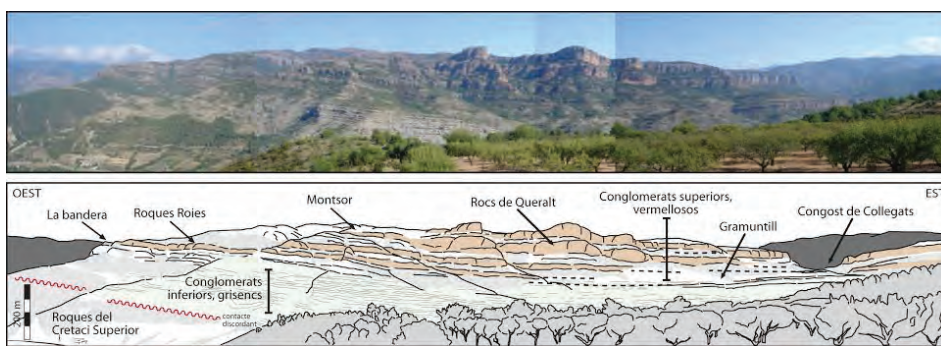
Vista panoràmica des del Torrent de Vallcarga fins a Collegats que mostra les dues famílies de conglomerats i la discordança amb la base cretàica. A la part baixa, els conglomerats grisençs. A la part mitjana, amb vegetació, el replà de Gramuntill, format per sediments dipositats en llacs. A la part alta, les capes de conglomerats vermellencs. Esquema cedit per Robert Duller (University of Liverpool, Regne Unit).
